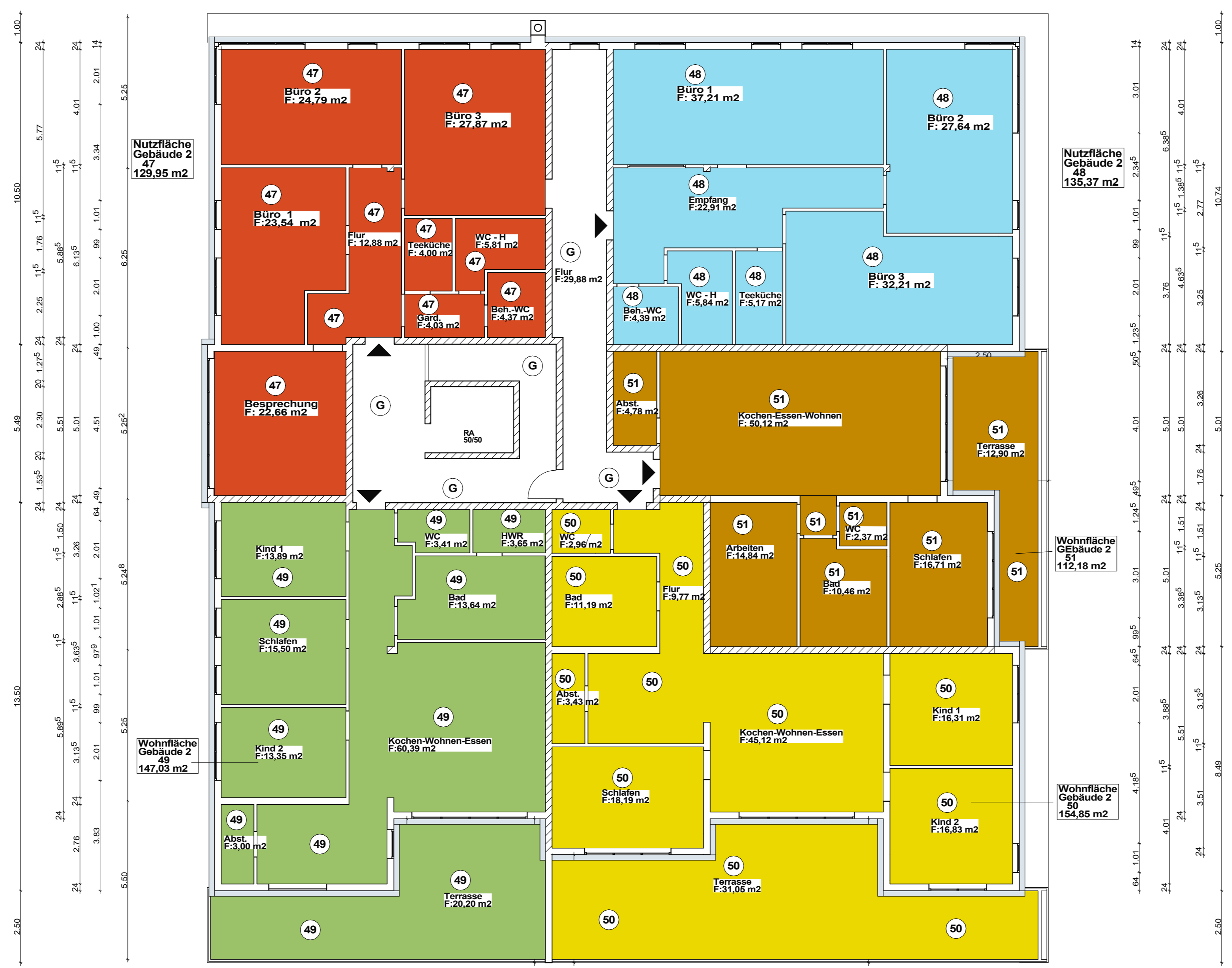
2. OBERGESCHOSS Gebäude 2
